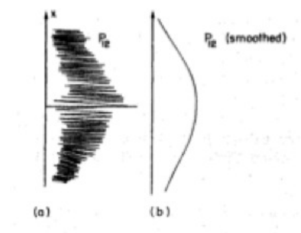
Figura 2.8: Esperimento delle due fenditure con i proiettili. Nella parte (a) è riportata l'immagine sullo schermo calcolata con la meccanica quantistica. Le rapide oscillazioni sono una rappresentazione della figura d'interferenza che si ottiene per lunghezze d'onda molto piccole. Ogni rivelatore fisicamente realizzabile, tuttavia, media le diverse oscillazioni di modo che la misura riproduce la curva continua riportata nella parte (b).
