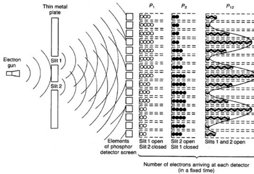
Figura 2.4: L'esperimento delle due fenditure eseguito con gli elettroni.
