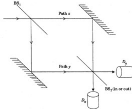
Figura 2.19: Schema di principio dell'interferometro Mach-Zender usato nell'esperimento di scelta ritardata. In questo caso entrambi gli specchi sono fissi, mentre BS_2 è mobile.
